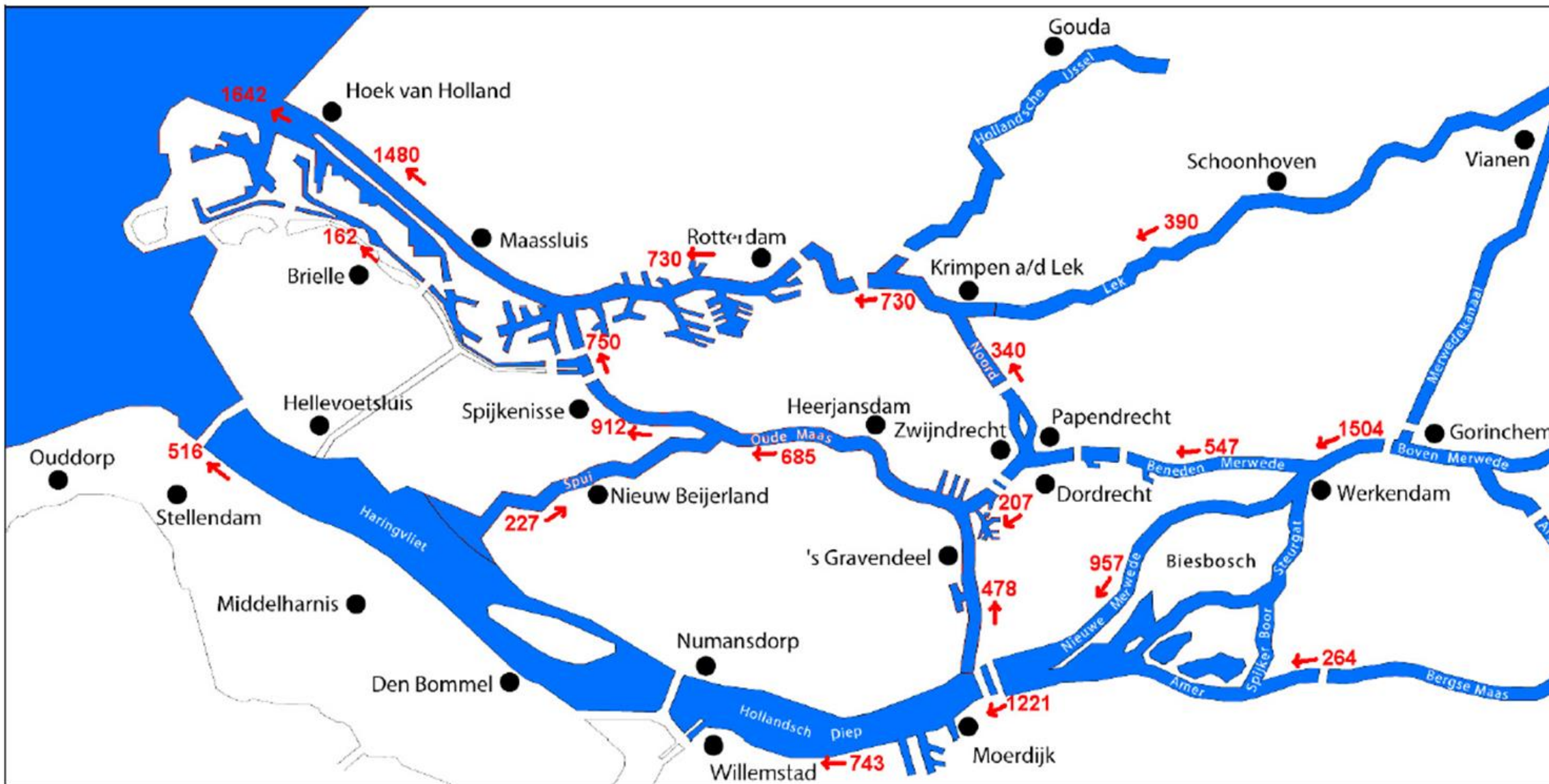
Figuur 9 (Netto)waterverdeling (in \text{m}^3/\text{s} ) bij een Bovenrijn afvoer van 2200 \text{ m}^3/\text{s} , bij gemiddeld getij (Hoek van Holland 1991.0). De verdeling is verkregen m.b.v. het model SOBEK, versie NDB1-0-0.
